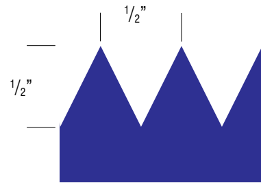
620310 1/2'' \times 1/2''
